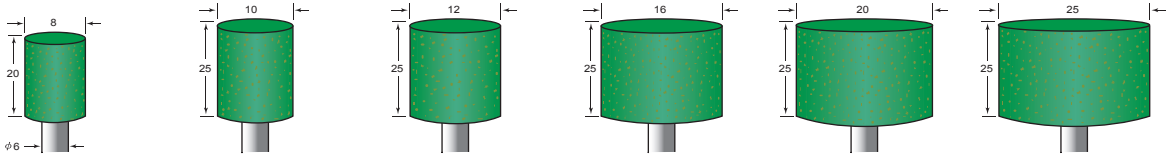
Cylinder 圓柱型
